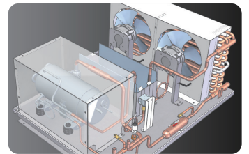
BLDC 인버터 적용 BLDC Inverter applied
