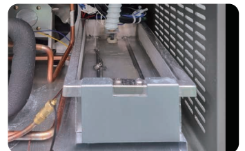
제상수 히터증발장치 Defrosting water heater evaporation device
